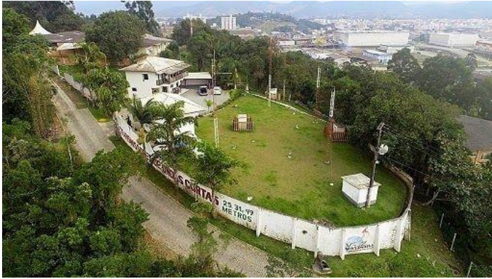
Het overzichtelijke antennenveld heeft een set van 3 dipolen, ontworpen voor hoog vermogen uitzendingen
